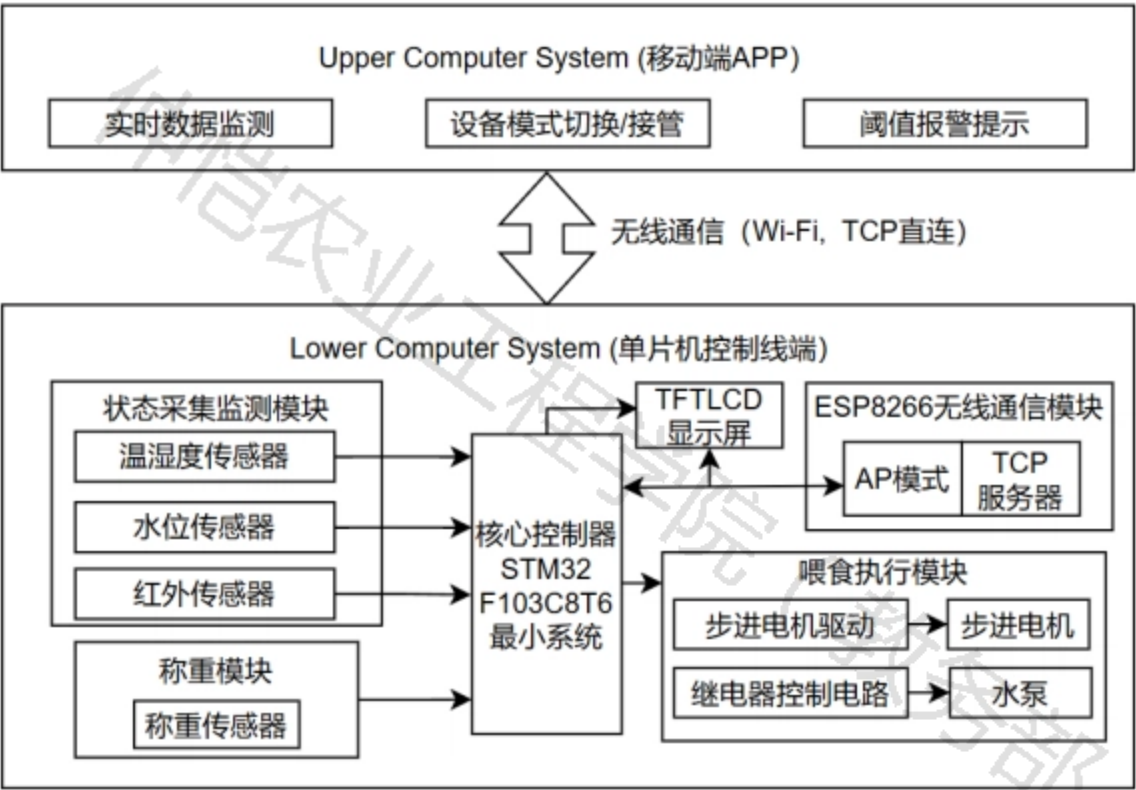
图1 系统框图
