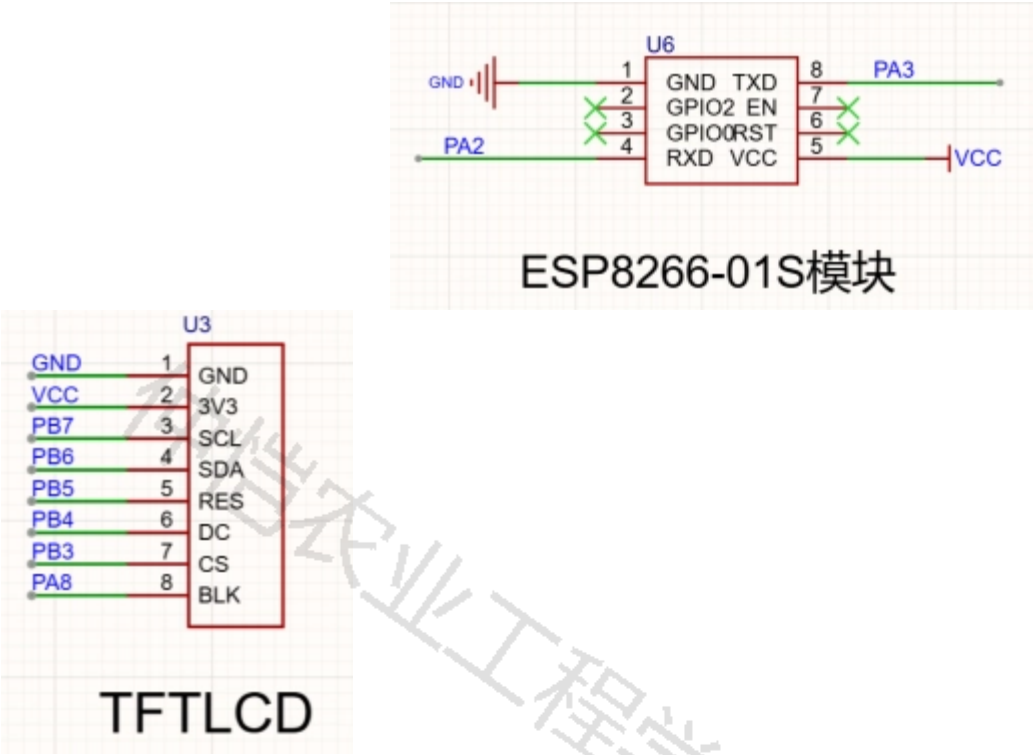
图20 通信与显示模块电路原理图
