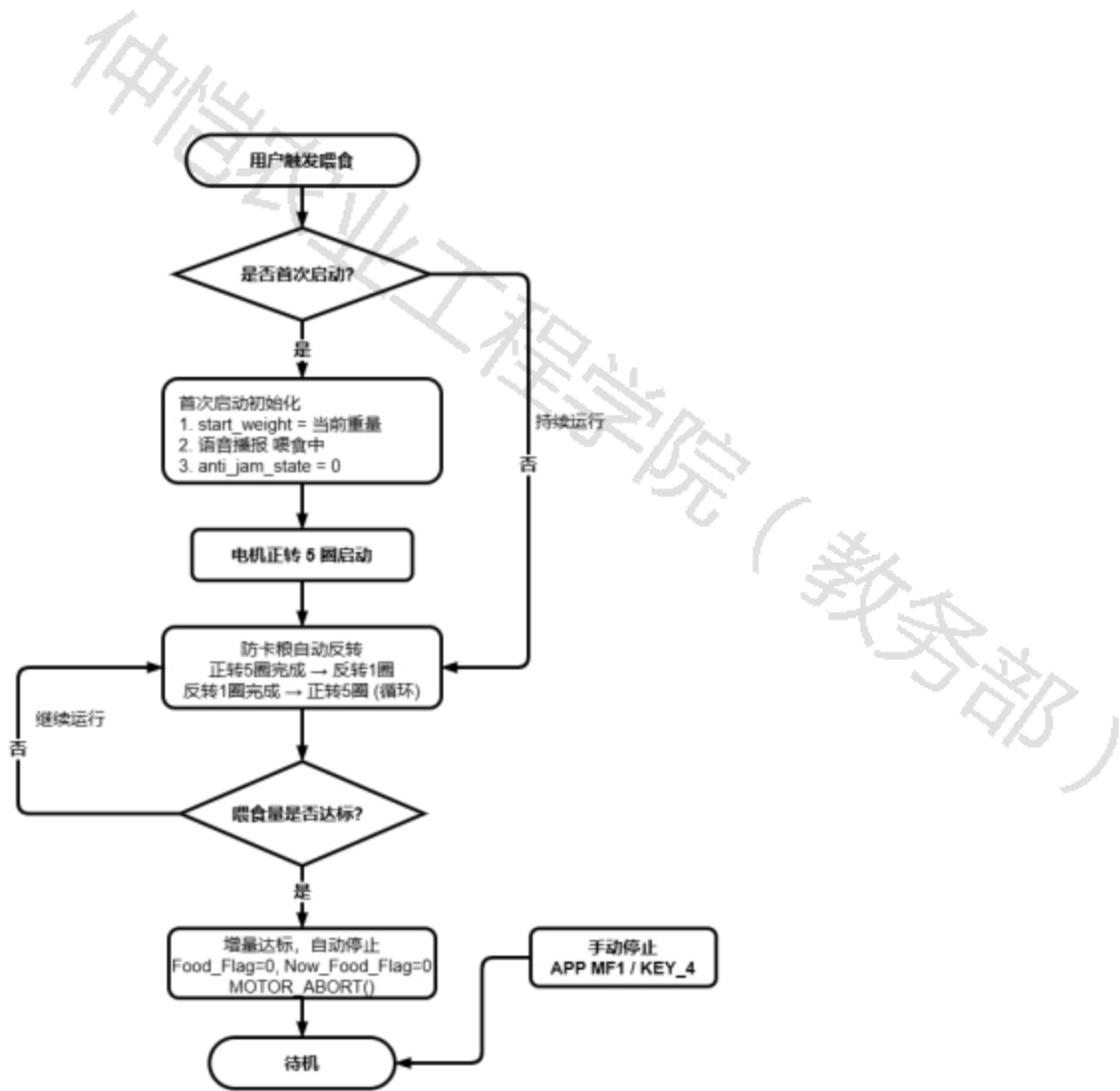
图22 智能喂食流程图
